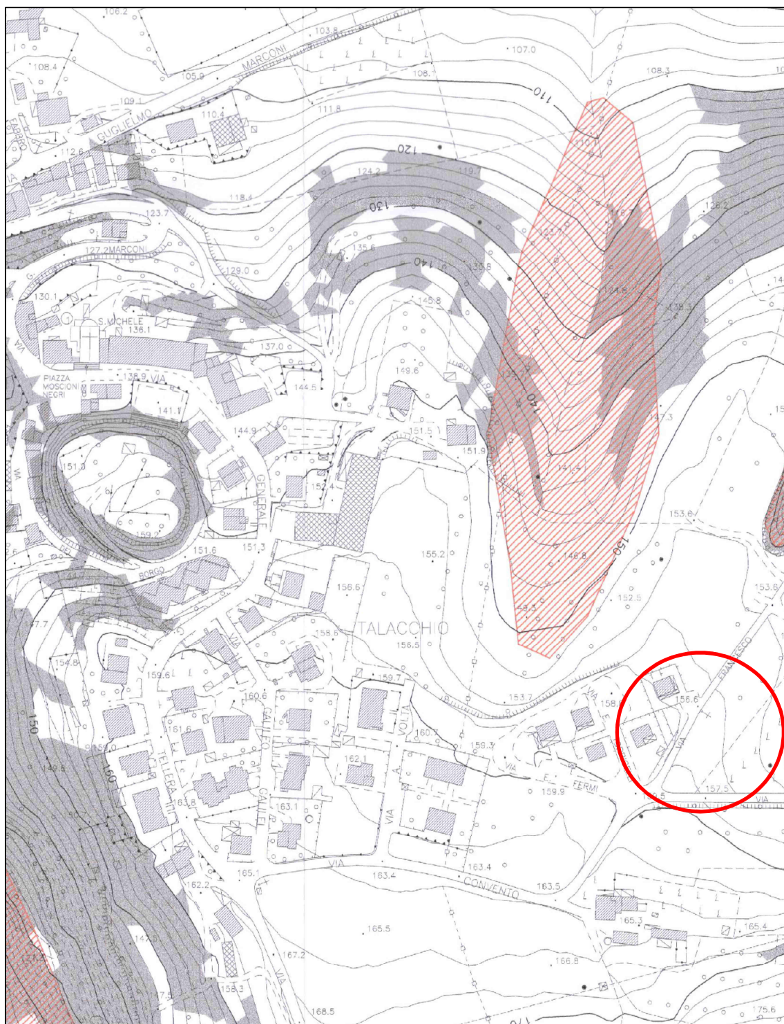
Figura 3-8 Stralcio Carta Pericolosità Sismiche ex comune di Colbordolo, la legenda è riportata in Appendice 1.
