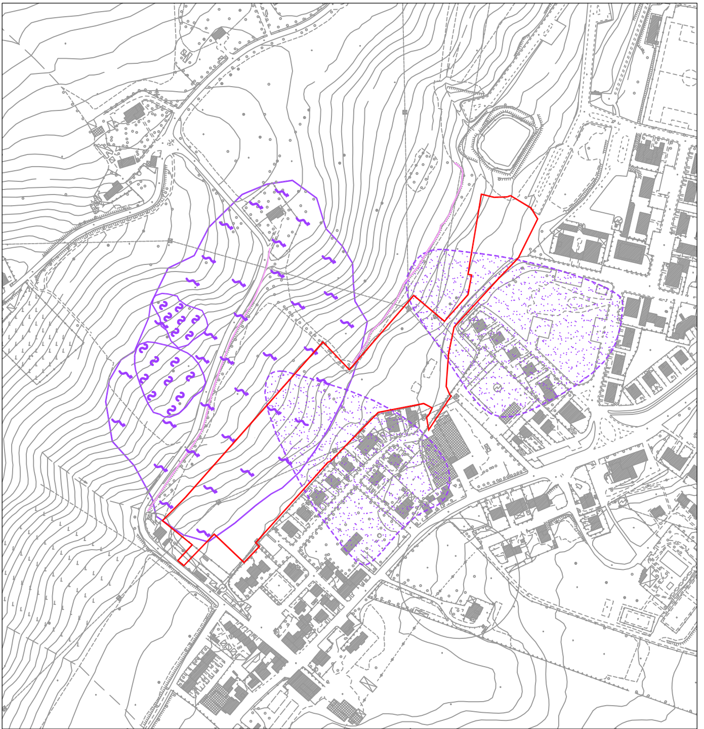
Carta di sintesi analisi fotogeologica - anno 1955
