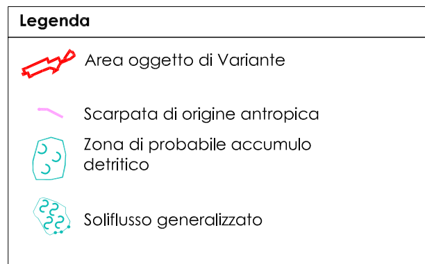
Carta di sintesi analisi fotogeologica - anno 2000
