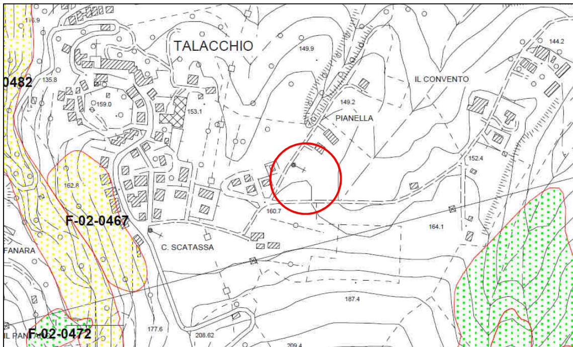
Figura 3-10 Stralcio Carta del Rischio Idrogeologico del Piano di Assetto Idrogeologico (P.A.I.) aggiornamento 2016.
