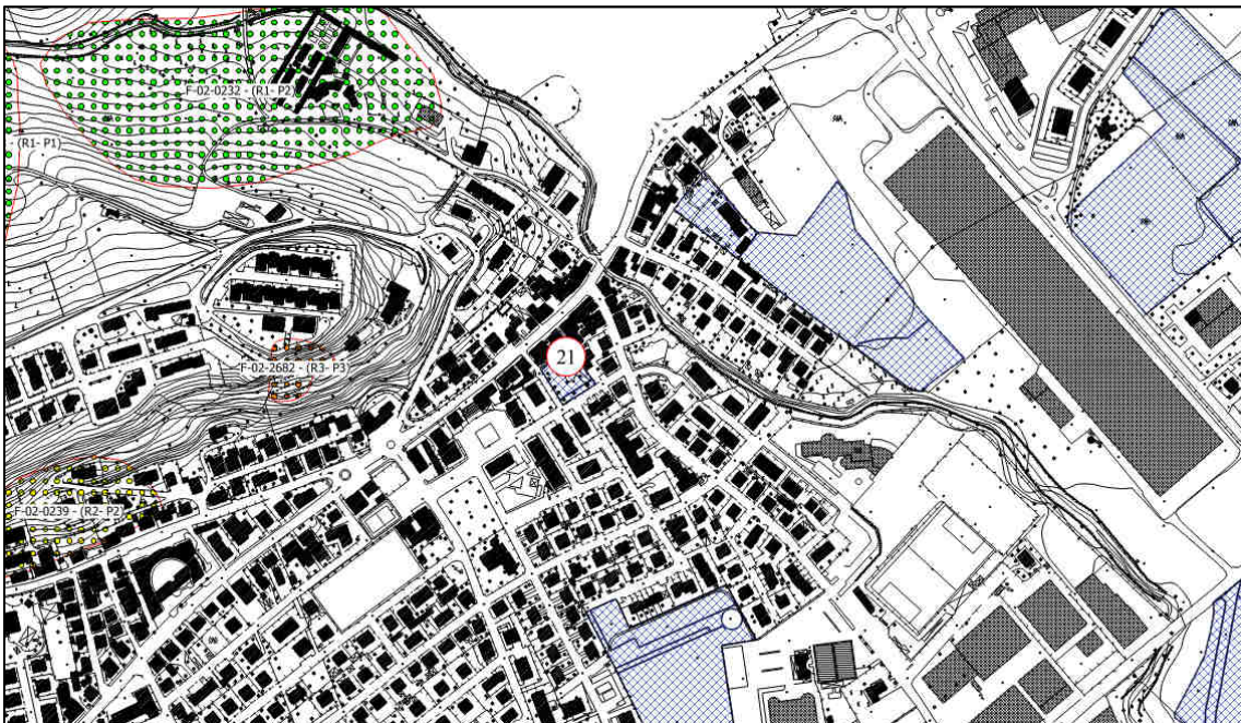
Figura 3-19 Stralcio Carta del Rischio Idrogeologico del Piano di Assetto Idrogeologico (P.A.I.) aggiornamento 2016 con evidenziata l'area interessata.
