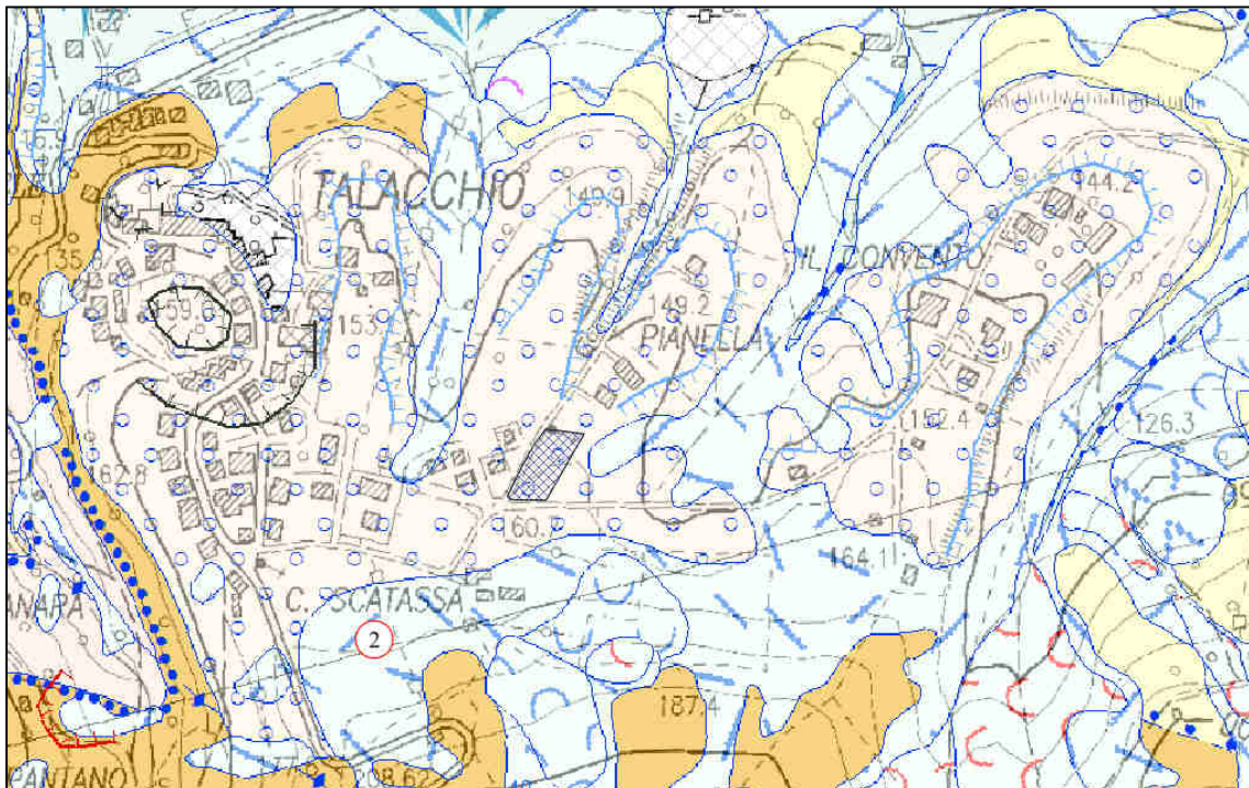
Figura 3-4 Stralcio CARG – la legenda è riportata in appendice alla presente relazione.
