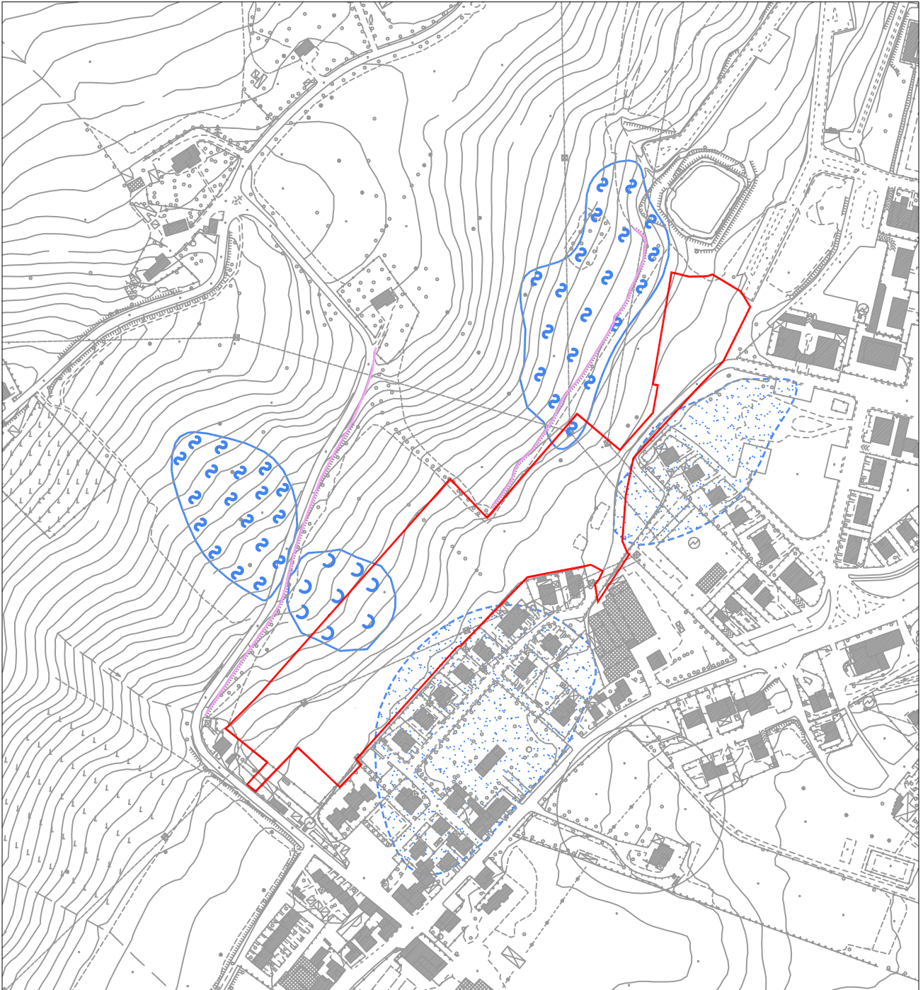
Carta di sintesi analisi fotogeologica - anno 1973
