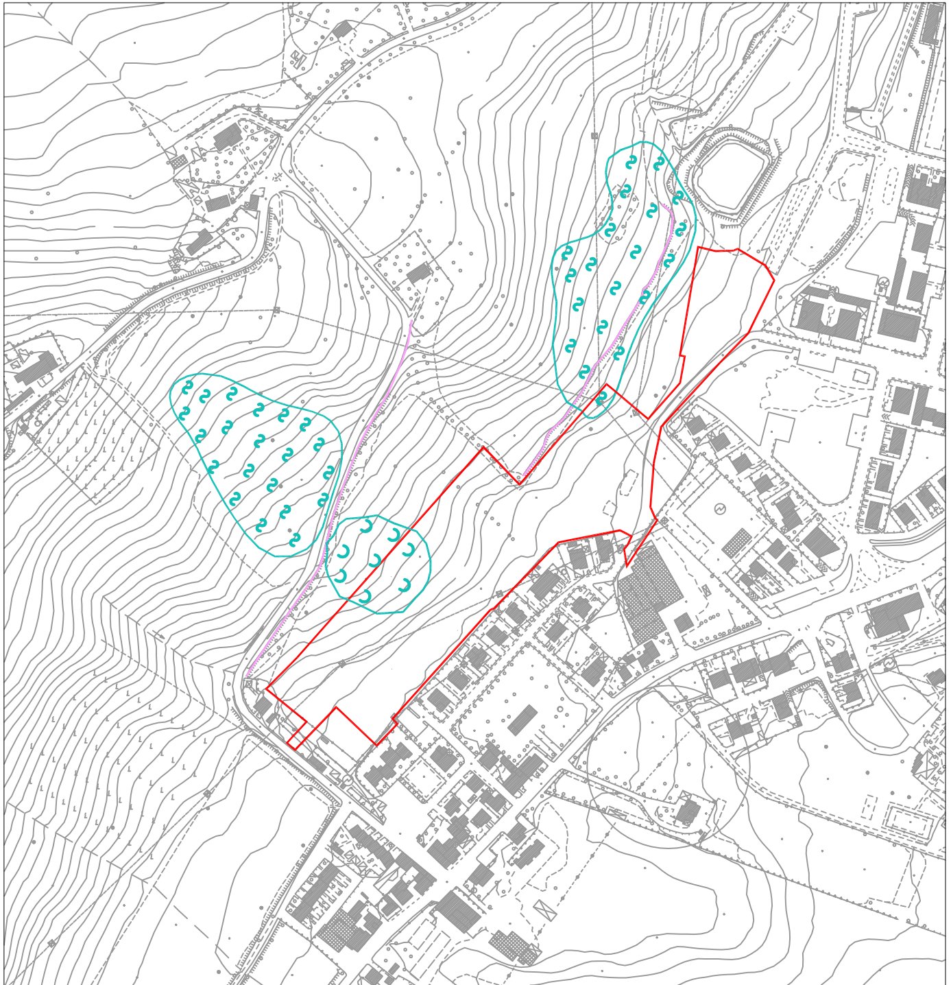
Carta di sintesi analisi fotogeologica - anno 2000
