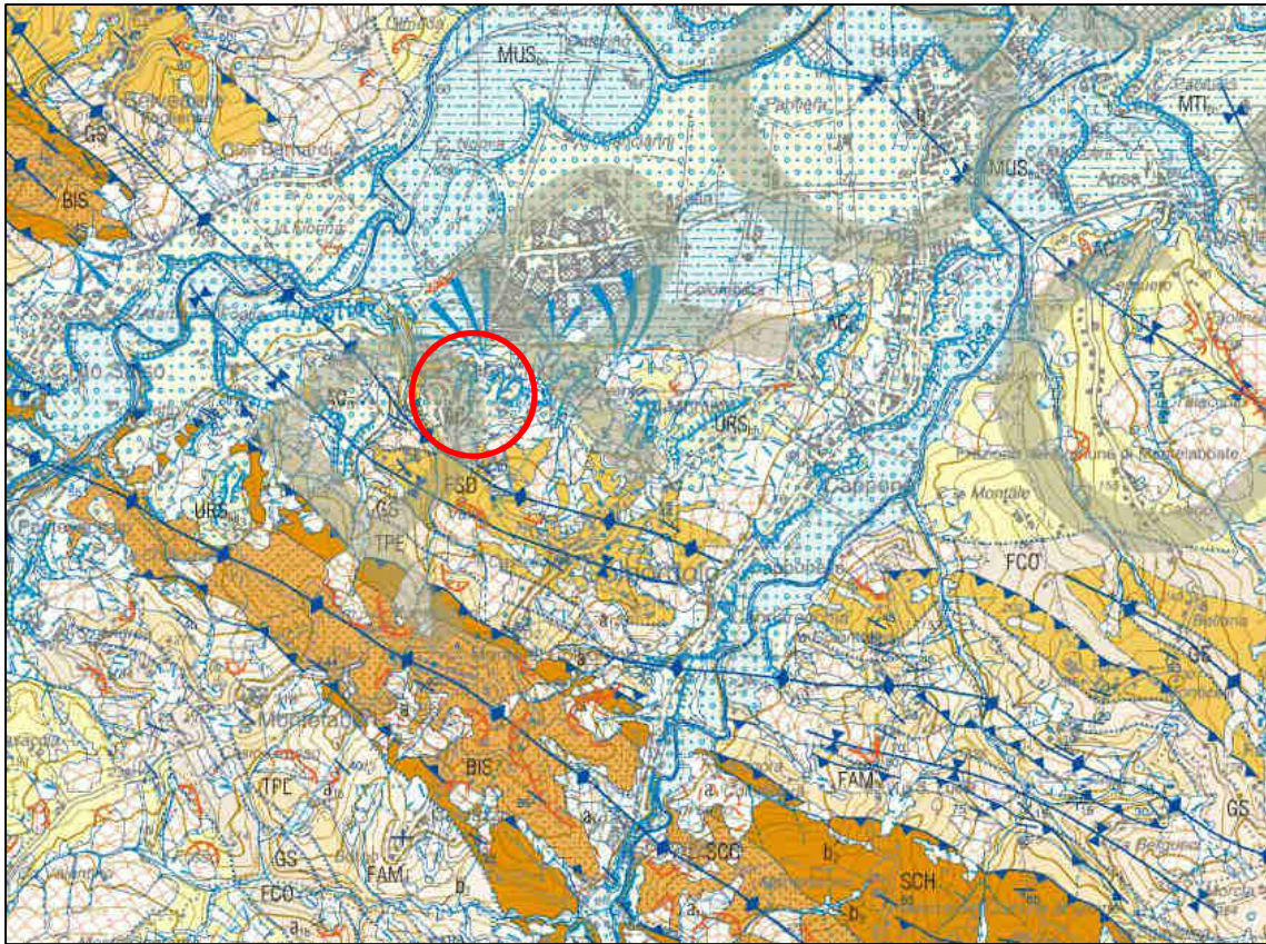
Figura 3-4 Stralcio CARG – la legenda è riportata in appendice alla presente relazione.
