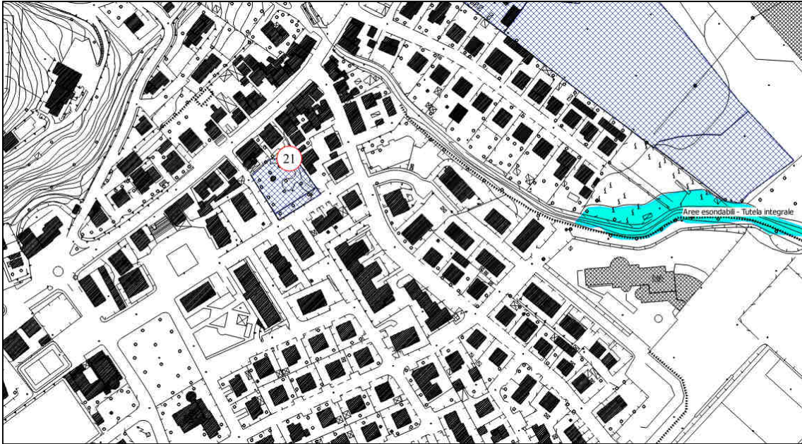
Figura 3-18 Stralcio del CTR con sovrapposizione dei tematismi di rischio idrogeologico riportati nelle nuove tavole di P.R.G. per l'area interessata.
