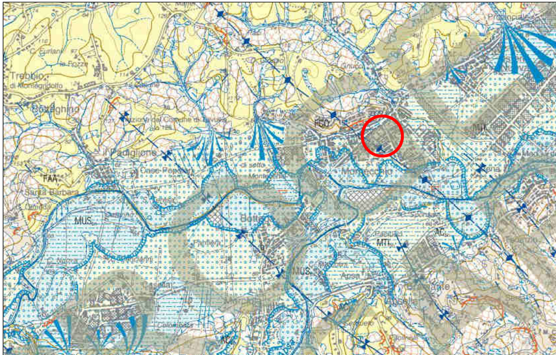
Figura 3-15 Stralcio Carta Geologica d'Italia Progetto CARG.
