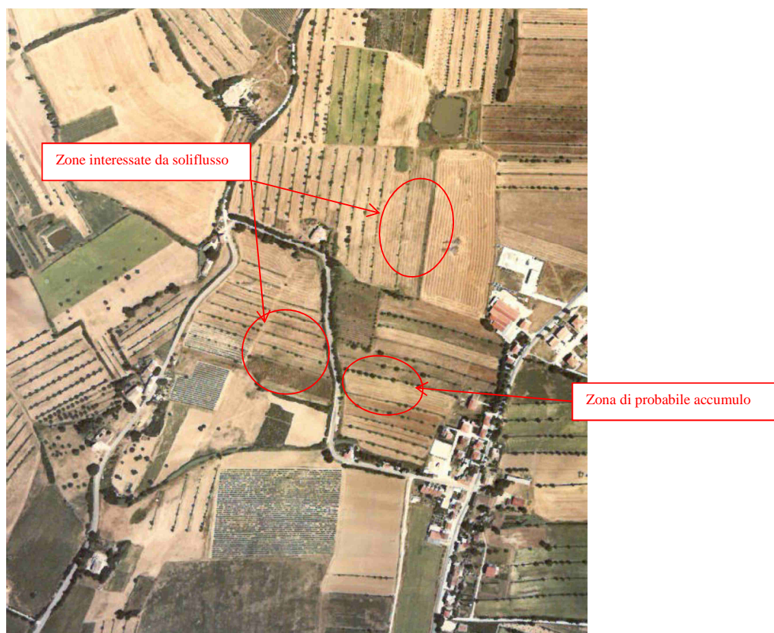
Figura 4-1 : Stralcio ingrandito foto aerea del 1973 – con evidenziate le aree interessate da soliflusso e l'area di accumulo detritico.
