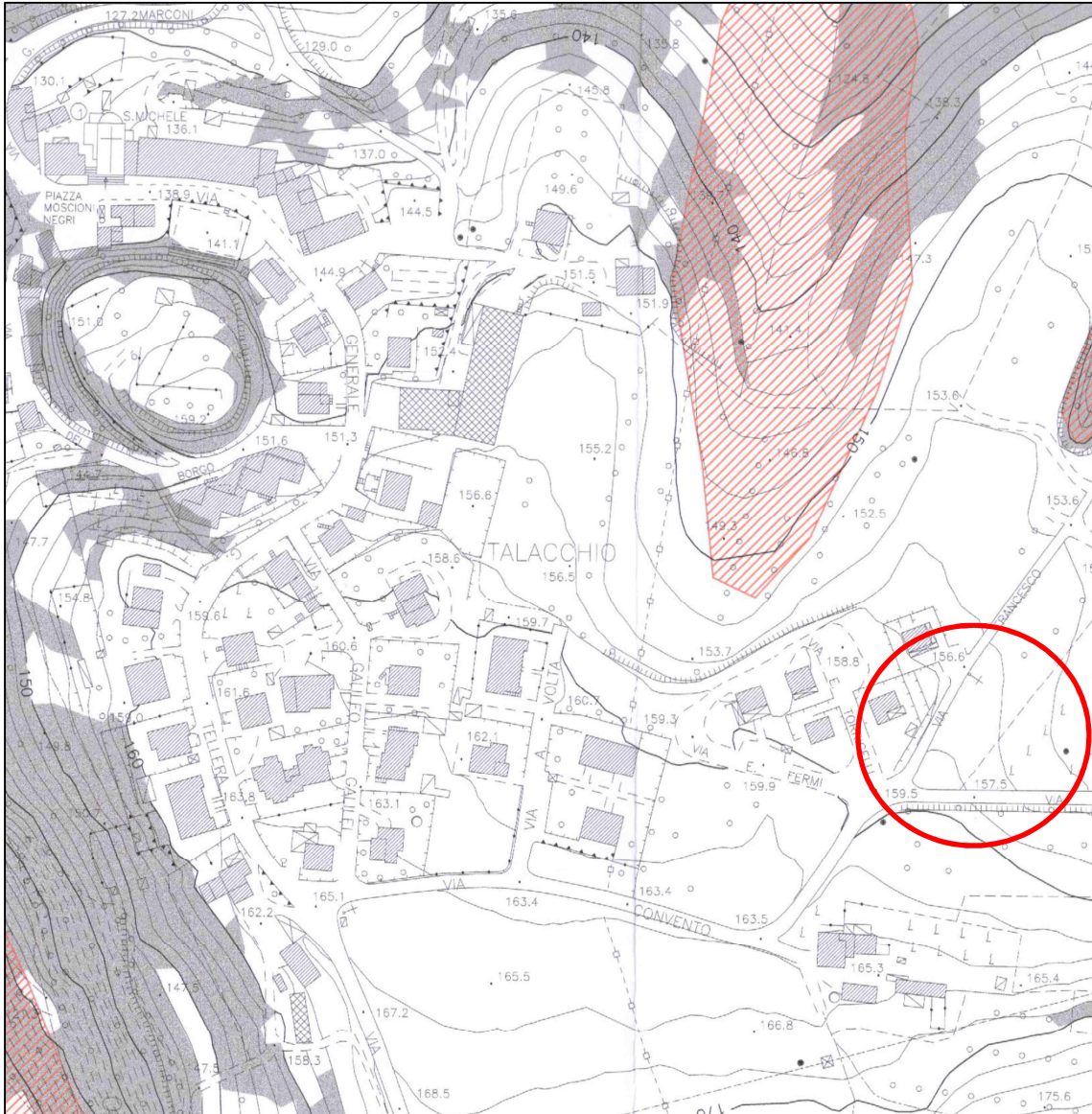
Figura 3-7 Stralcio Carta Geomorfológica ex comune di Colbordolo, la legenda è riportata in Appendice 1.
