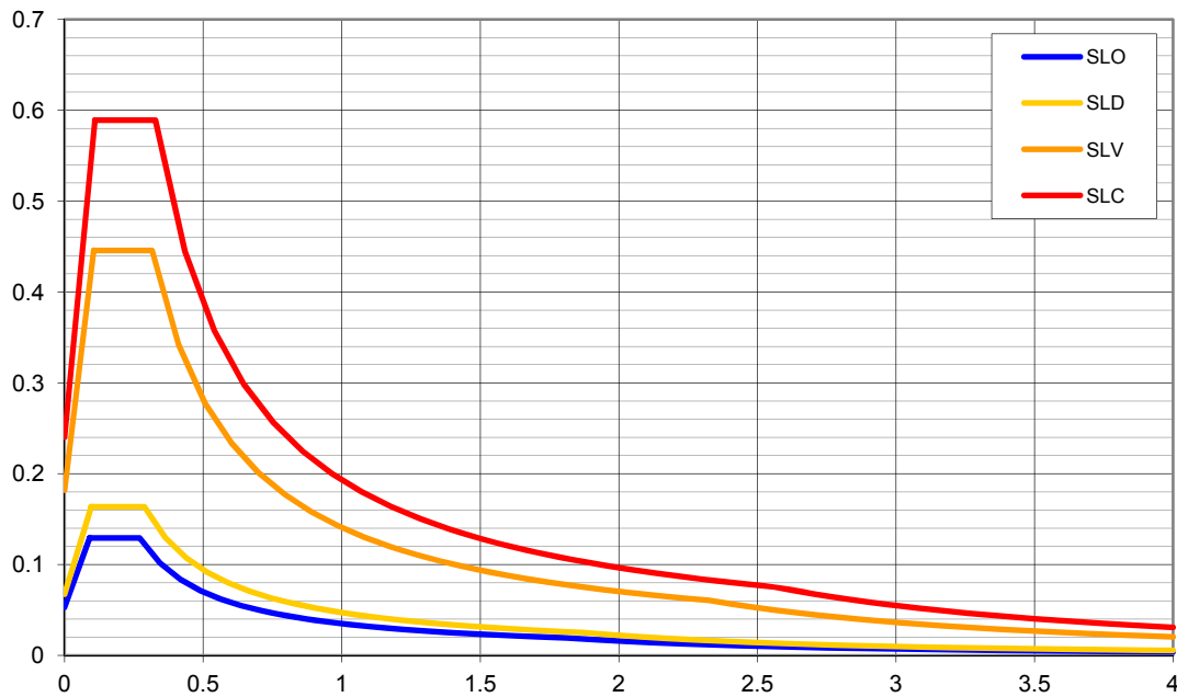
Figura 4.1: Spettri di risposta elastici normalizzati per i diversi Stati Limite riferiti ad un suolo rigido e ad una topografia orizzontale (cat. A – T1 da NTC 2018).
