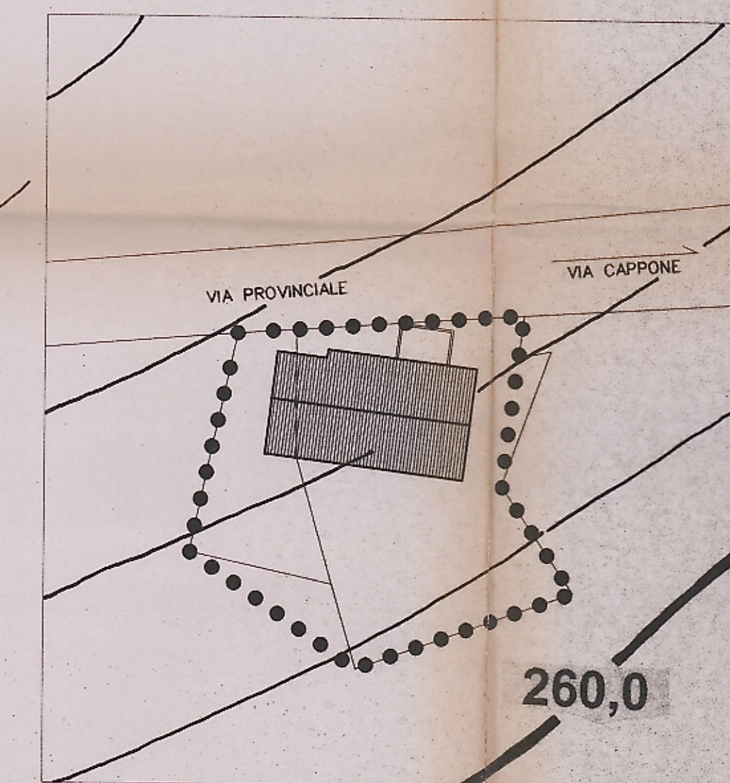
PARTICOLARE B
