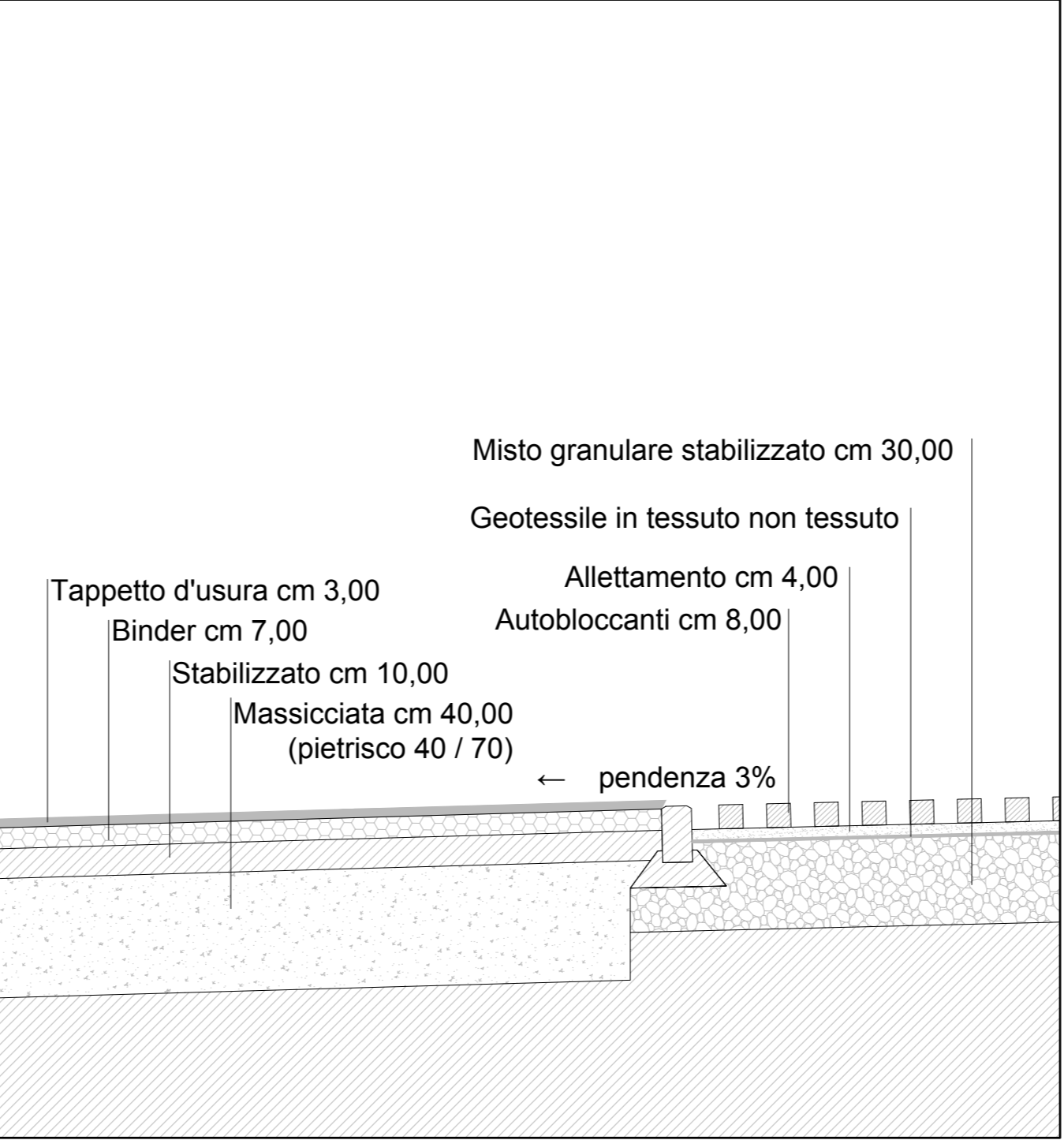
PARTICOLARI COSTRUTTIVI STRADA E PARCHEGGI Scala 1:20
