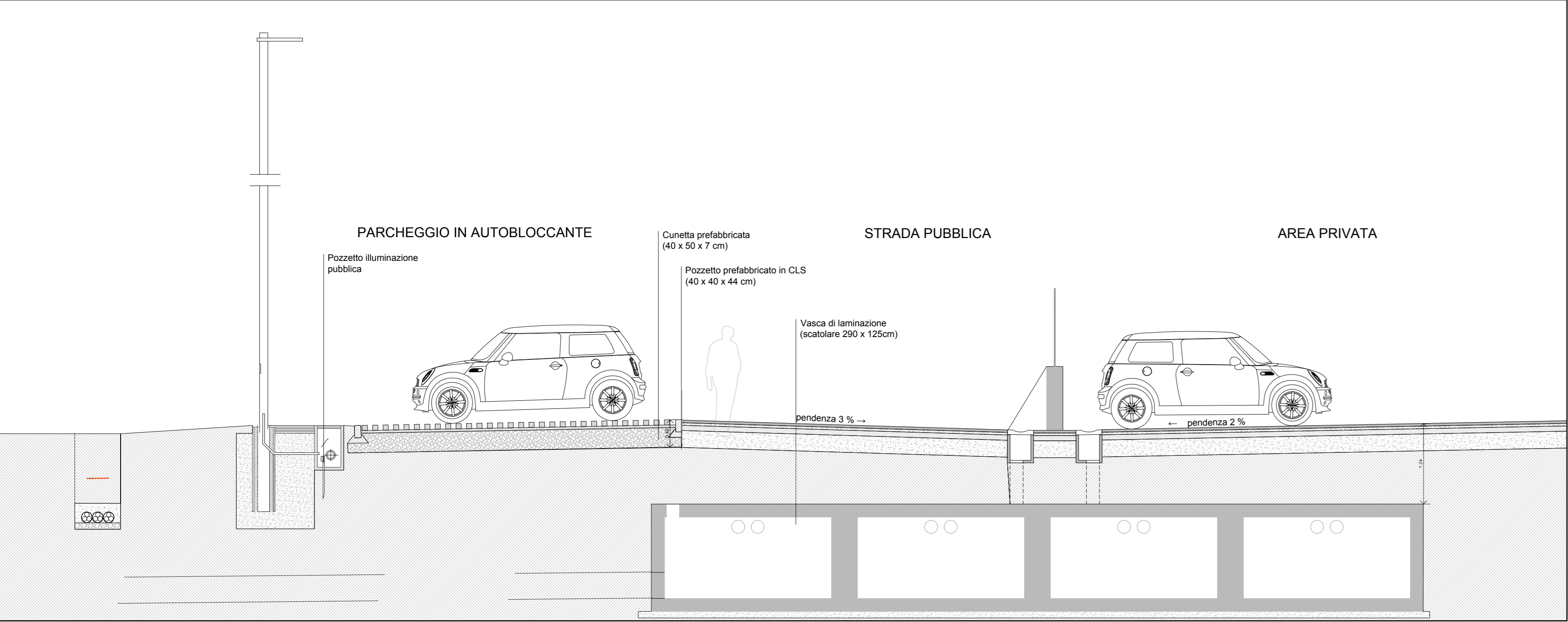
SEZIONE STRADALE A-A Scala 1:50
