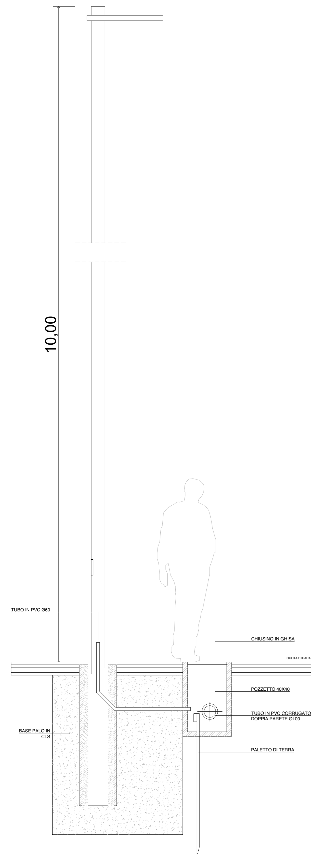
DETTAGLI COSTRUTTIVI CORPI ILLUMINANTI - SCALA 1:20
